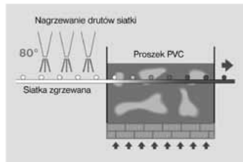
Fluidyzacja (sintercoating)
